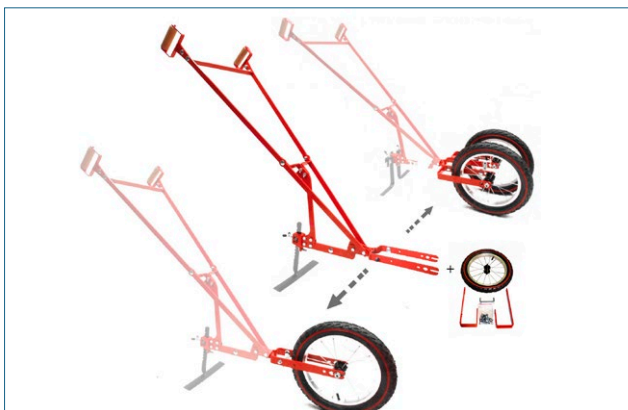
Bild 1. Med ett enkelt handgrepp byggs enhjulshackan om till tvåhjulshacka – eller tvärt om.
